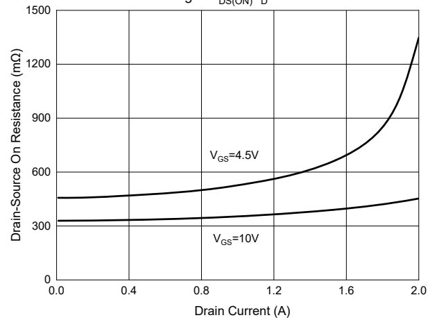
Fig.4- R_{DS(ON)}-I_D
