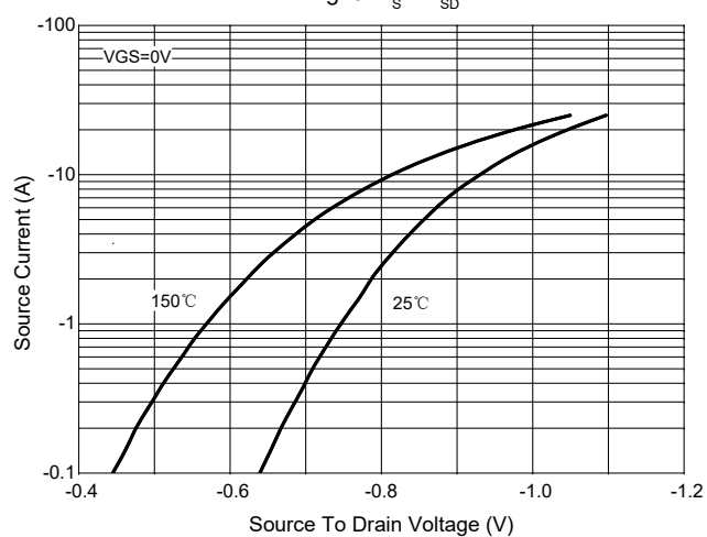
Fig. 9 - I_S - V_{SD}
