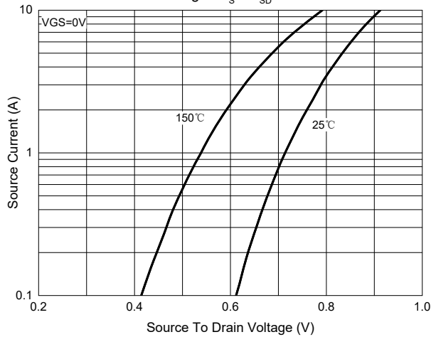
Fig.9 - I_S - V_{SD}
