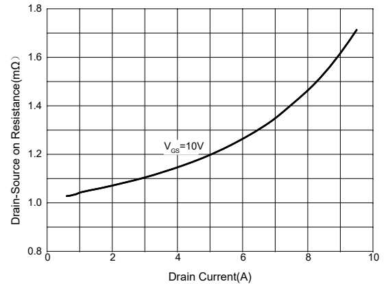
Fig. 4 - R_{DS(ON)} - I_D
