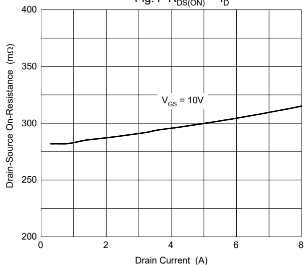
Fig.4- R_{DS(ON)} - I_D
