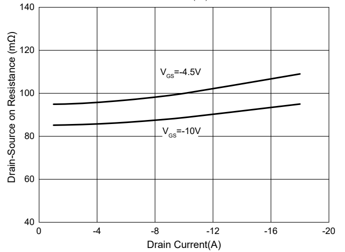
Fig. 4 - R_{DS(ON)} - I_D
