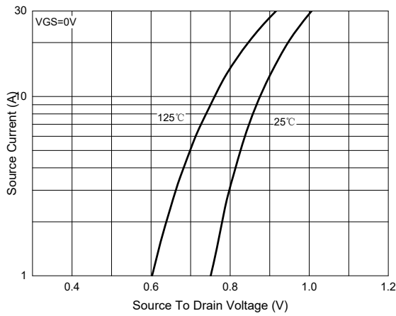
Fig.9 - I_S - V_{SD}
