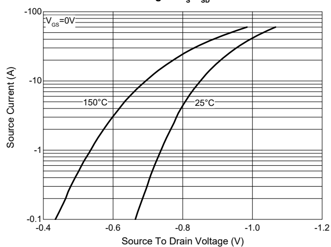
Fig. 9 - I_S - V_{SD}
