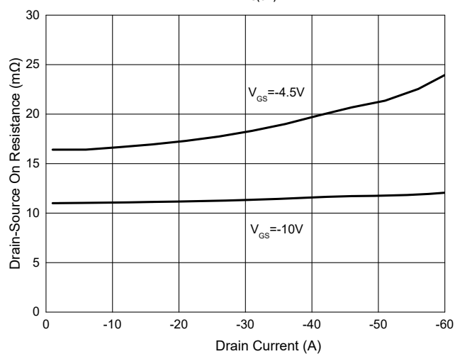
Fig. 4 - R_{DS(ON)} - I_D
