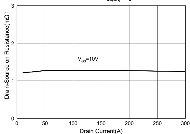
Fig. 4 - R_{DS(ON)} - I_D
