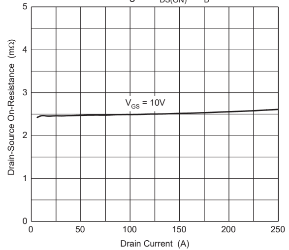
Fig.4- R_{DS(ON)} - I_D
