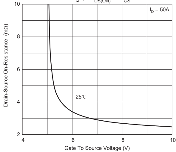
Fig.3- R_{DS(ON)} - V_{GS}
