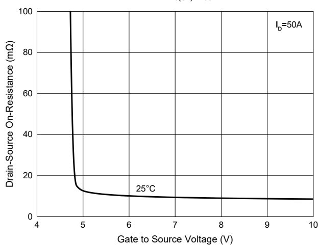
Fig. 3 - R_{DS(ON)} - V_{GS}
