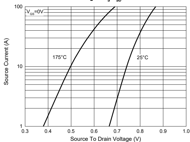
Fig. 9 - I_S - V_{SD}
