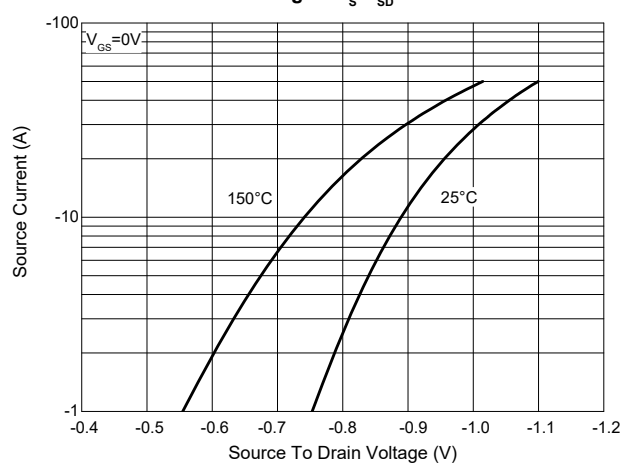
Fig. 9 - I_S - V_{SD}
