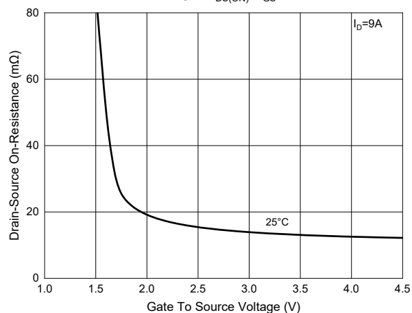
Fig.3- R_{DS(ON)}-V_{GS}
