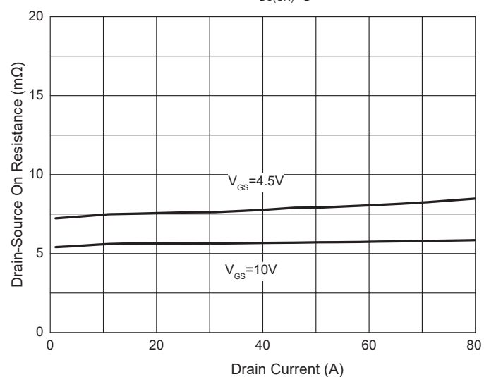
Fig. 4 - R_{DS(ON)} - I_D
