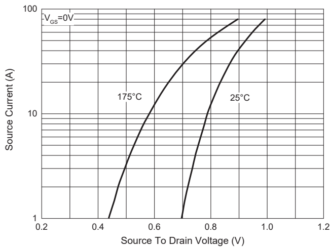
Fig. 9 - I_S - V_{SD}
