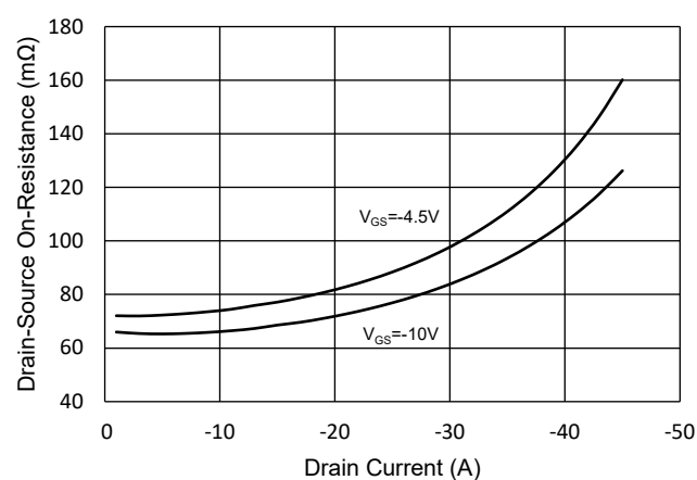
Fig.4 - R_{DS(ON)} - I_D
