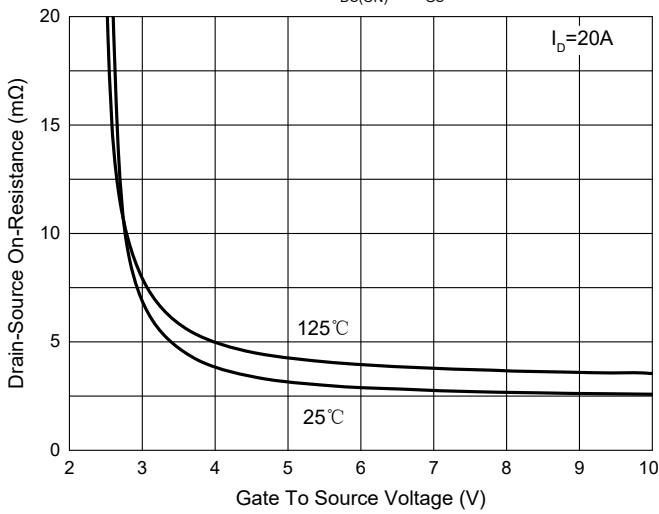
Fig. 3 - R_{DS(ON)} - V_{GS}
