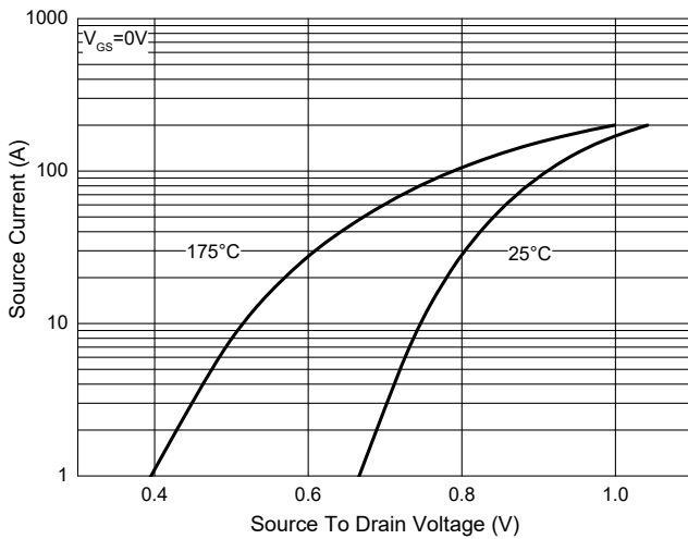
Fig. 9 - I_S - V_{SD}
