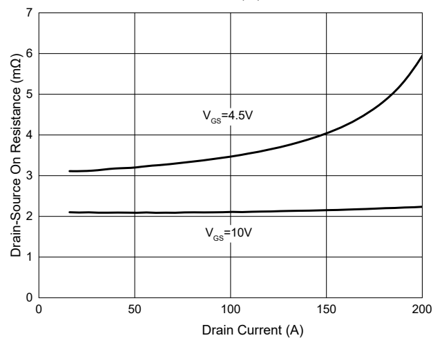
Fig. 4 - R_{DS(ON)} - I_D
