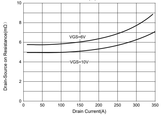
Fig. 4 - R_{DS(ON)} - I_D
