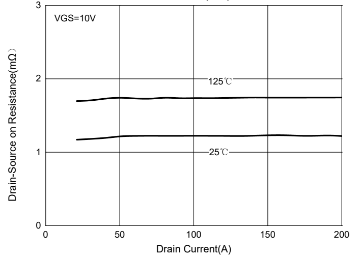
Fig. 4 - R_{DS(ON)} - I_D
