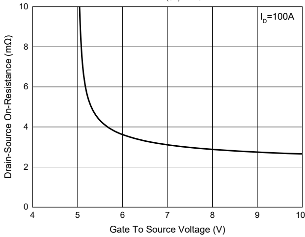
Fig. 3 - R_{DS(ON)} - V_{GS}
