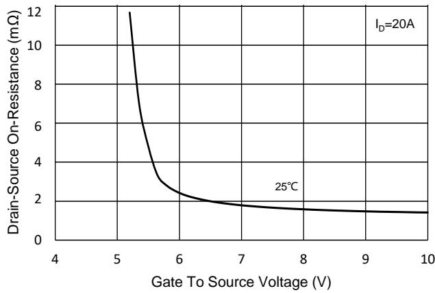
Fig.3 - R_{DS(ON)} - V_{GS}
