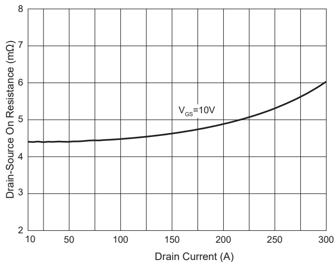
Fig. 4 - R_{DS(ON)}-I_D
