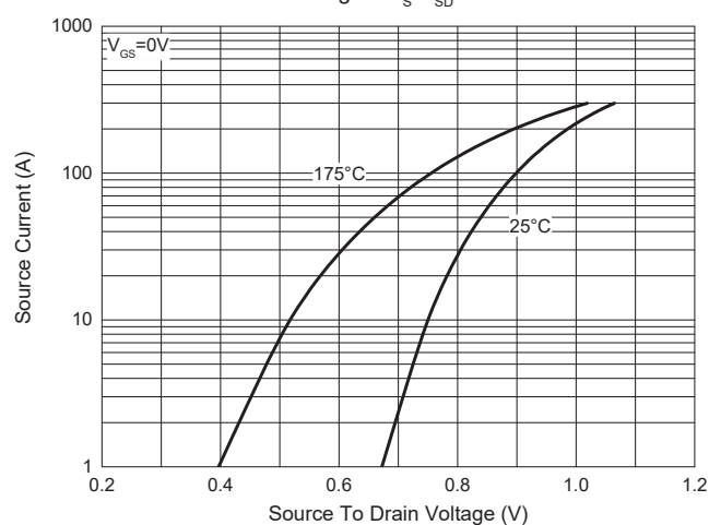
Fig. 9 - I_S - V_{SD}
