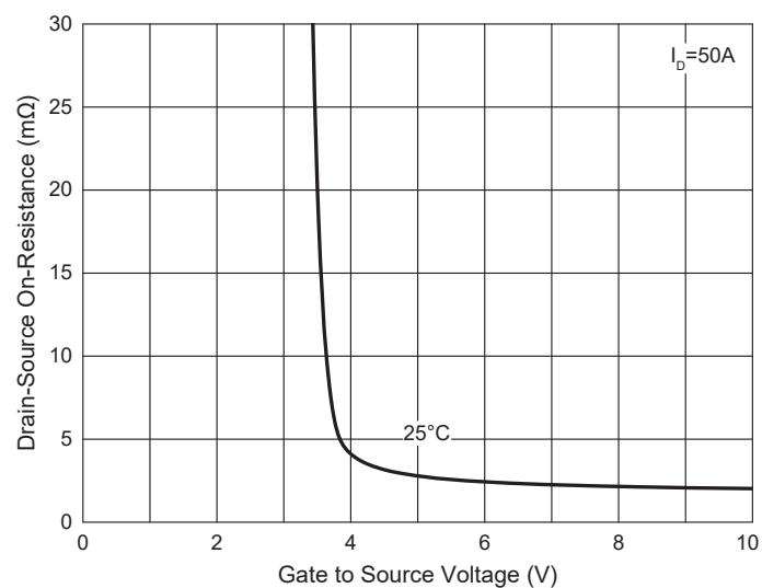
Fig. 3 - R_{DS(ON)} - V_{GS}
