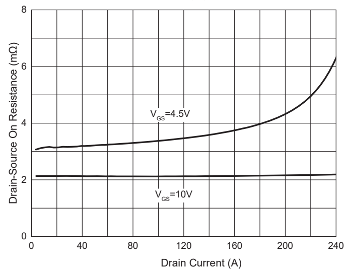
Fig. 4 - R_{DS(ON)} - I_D
