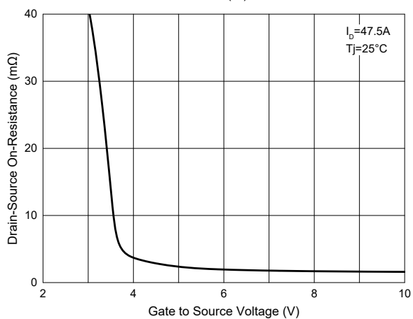
Fig. 3 - R_{DS(ON)} - V_{GS}
