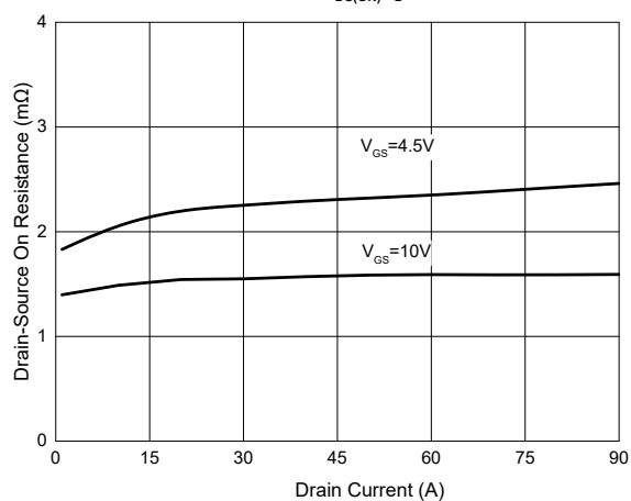
Fig. 4 - R_{DS(ON)} - I_D
