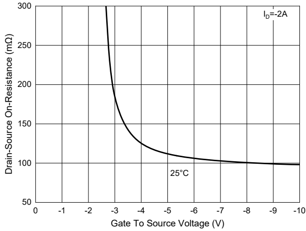
Fig.3- R_{DS(ON)} - V_{GS}
