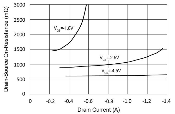
Fig.4 - R_{DS(ON)} - I_D
