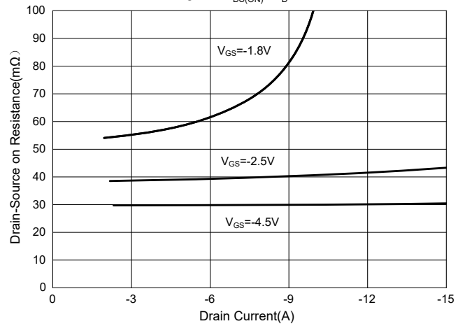
Fig. 4 - R_{DS(ON)} - I_D
