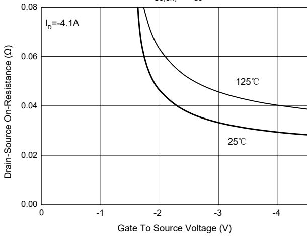
Fig. 3 - R_{DS(ON)} - V_{GS}
