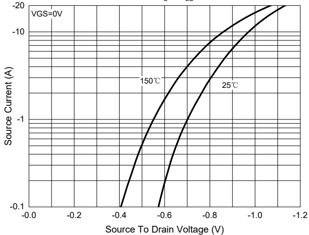
Fig.9 - I_s - V_{SD}
