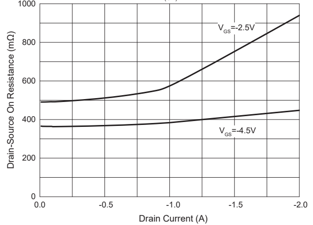
Fig.4- R_{DS(ON)}-I_D
