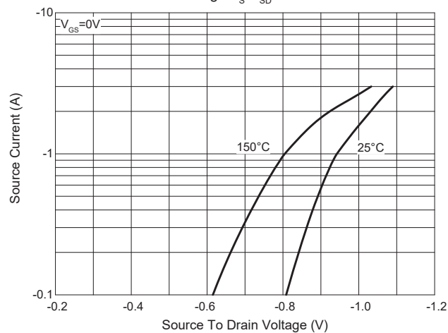
Fig.9- I_S - V_{SD}
