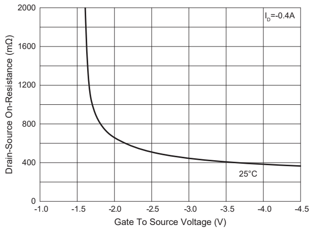
Fig.3- R_{DS(ON)}-V_{GS}
