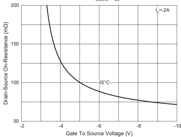
Fig.3- R_{DS(ON)} - V_{GS}
