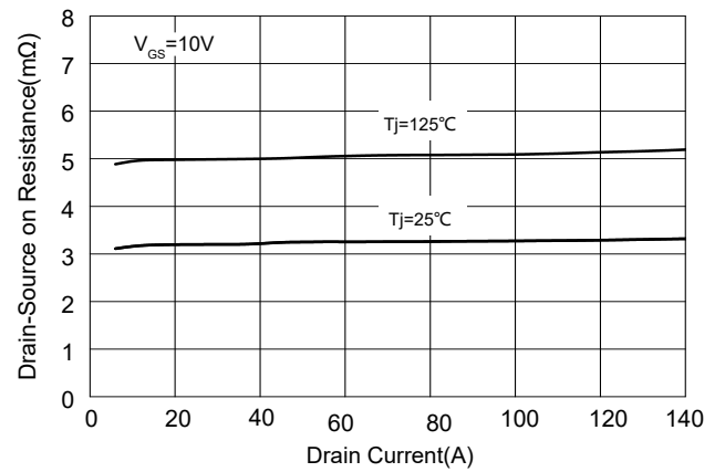
Fig.4 - R_{DS(ON)} - I_D
