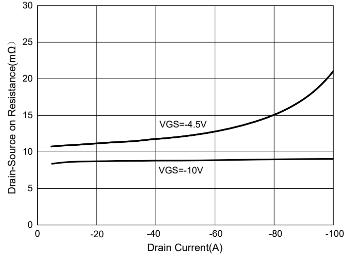
Fig. 4 - R_{DS(ON)} - I_D
