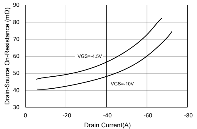
Fig.4 RDS(ON)-ID
