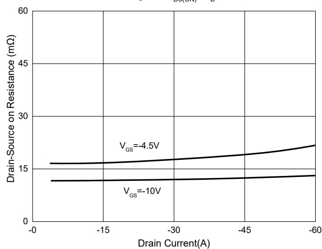
Fig. 4 - R_{DS(ON)} - I_D
