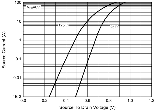
Fig.9 - I_S - V_{SD}
