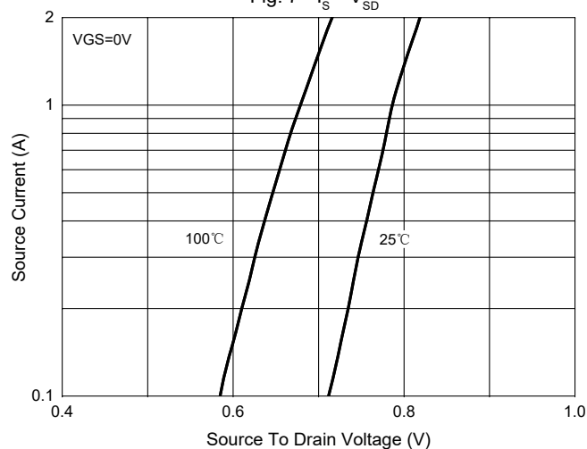
Fig. 7 - I_s - V_{SD}
