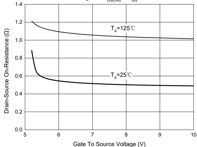
Fig. 4 - R_{DS(ON)} - V_{GS}
