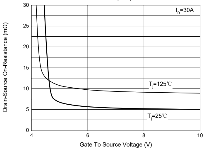
Fig. 3 - R_{DS(ON)} — V_{GS}
