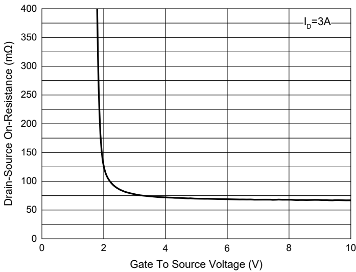
Fig. 3 - R_{DS(ON)} - V_{GS}
