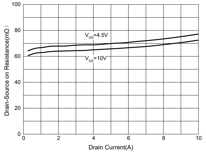
Fig. 4 - R_{DS(ON)} - I_D
