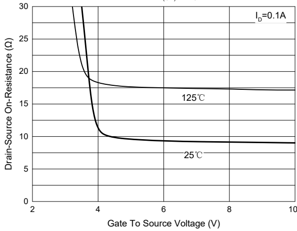
Fig. 3 - R_{DS(ON)} - V_{GS}
