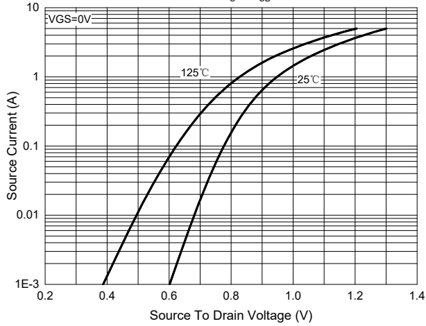
Fig.9 - I_s - V_{SD}
