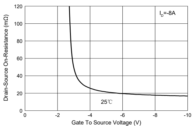
Fig.3 - R_{DS(ON)} - V_{GS}
