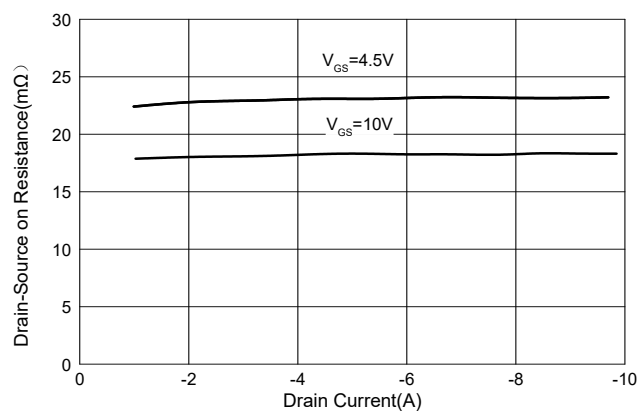
Fig.4 - R_{DS(ON)} - I_D
