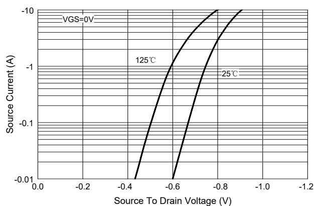
Fig.9 - I S - V SD
