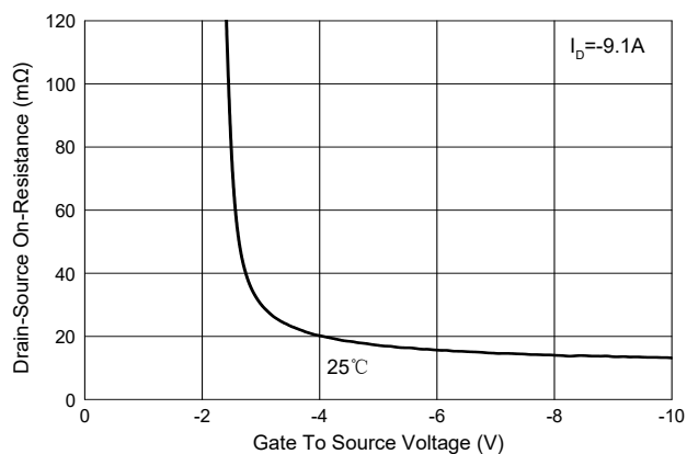
Fig.3 - R_{DS(ON)} - V_{GS}
