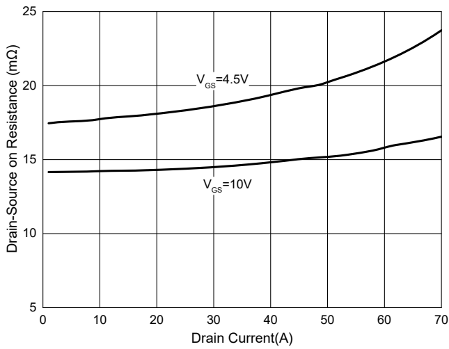
Fig. 7 - R_{DS(ON)} - I_D
