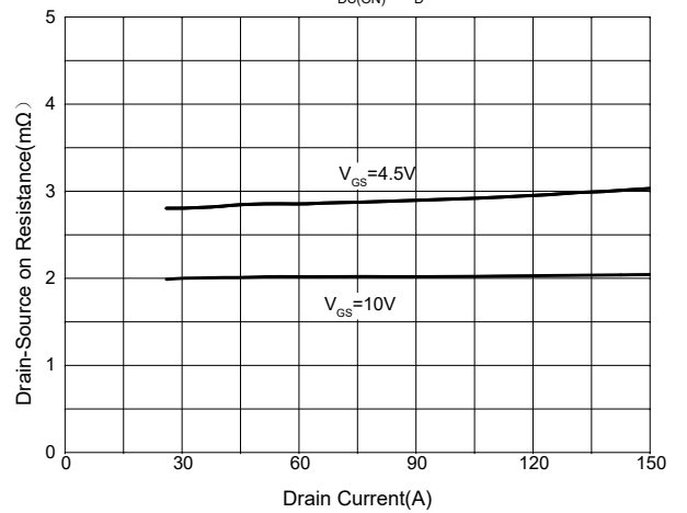
Fig. 4 - R_{DS(ON)} - I_D
