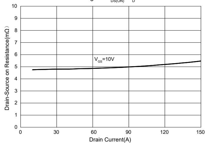
Fig. 4 - R_{DS(ON)} - I_D
