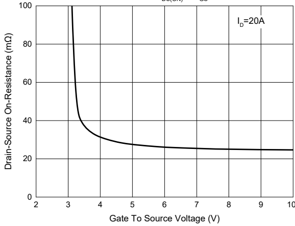
Fig. 3 - R_{DS(ON)} - V_{GS}
