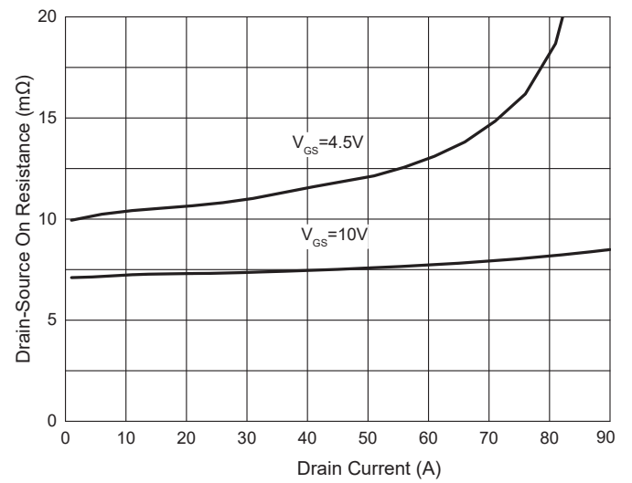
Fig. 4 - R_{DS(ON)} - I_D
