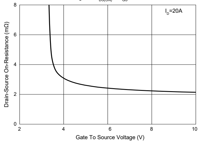
Fig. 3 - R_{DS(ON)} - V_{GS}
