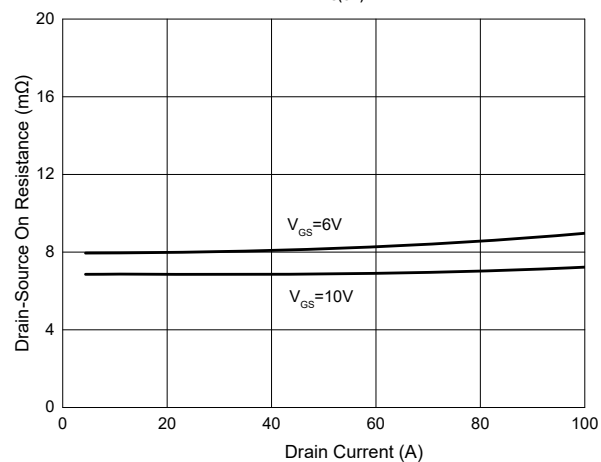
Fig. 4 - R_{DS(ON)} - I_D
