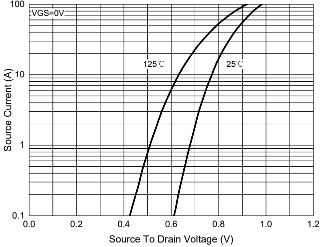
Fig.9 - I_S - V_{SD}
