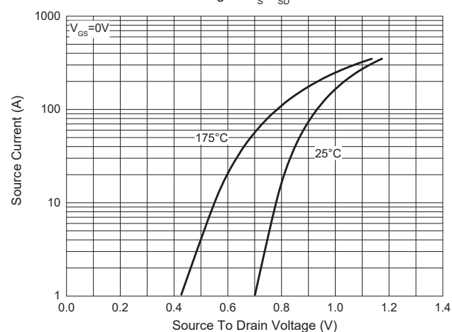
Fig. 9 - I_S - V_{SD}
