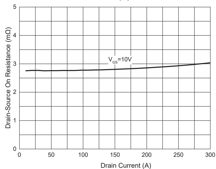
Fig. 4 - R_{DS(ON)} - I_D
